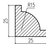
Ćwierćwałek wypukły 25x25
