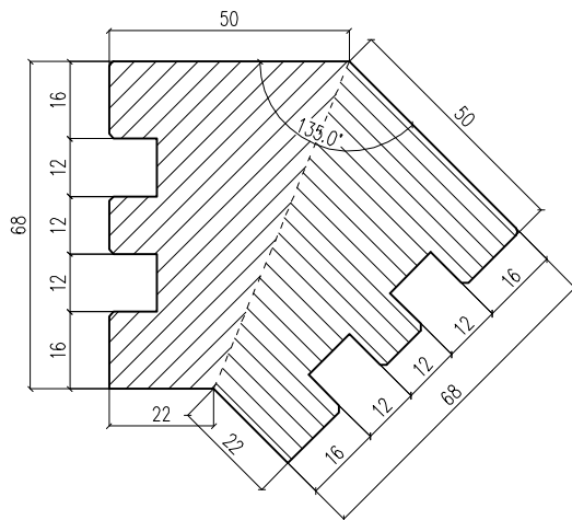
Belka narożna 135°
